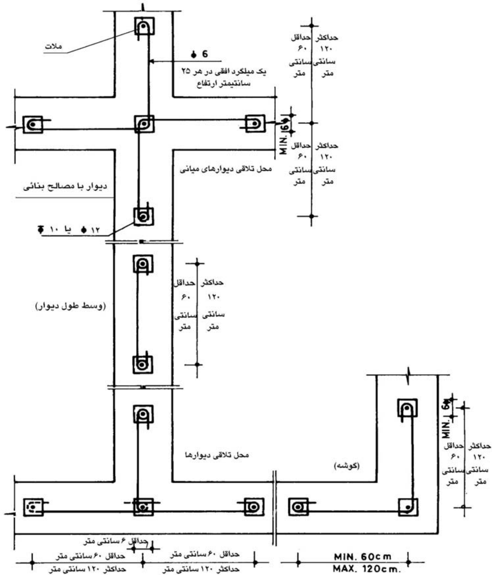
شکل (۸-۱): جزئیات میلگردهای قائم و افقی مهارت دیوارها.
